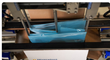
4 Allargamento del soffietto della busta
